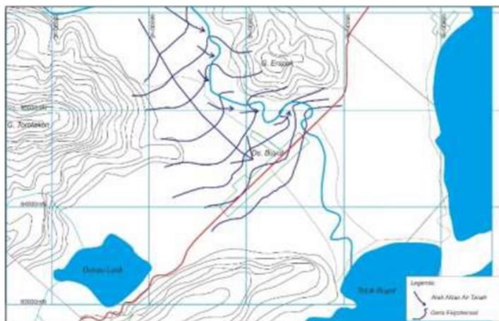
Gambar 4. Sistem akifer bebas desa Buyat
