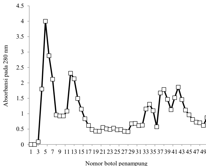
Gambar 3. Profil fraksi dari kromatografi kolom yang dibaca pada λ 280 nm
