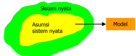
Gambar 1. Abstraksi pemodelan Sumber : Taha, 1992.
