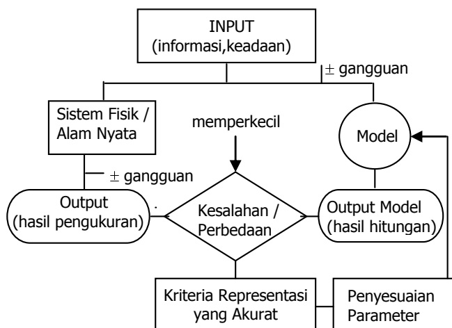
Gambar 4. Konsep model matematik Sumber : Fleming, 1975.
