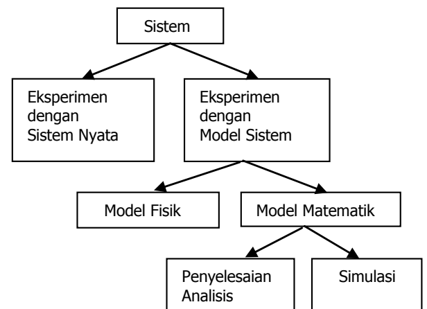
Gambar 2. Klasifikasi pemodelan sistem Sumber : Law dan Kelton, 1991.
