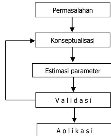
Gambar 3. Proses Pemodelan Sumber : Rinaldi dkk, 1979.
