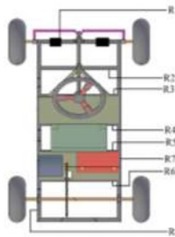
Gambar 4.4 Tampak Atas Gokar
