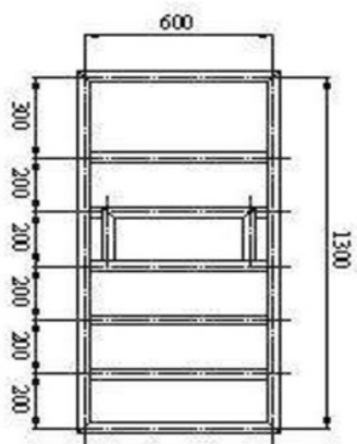
TAMPAK ATAS
