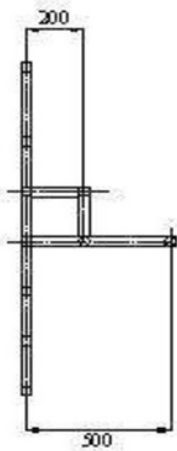
TAMPAK DEPAN
