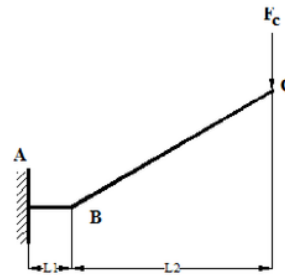
Gambar 3 Pembebanan pada poros Landing Gear
