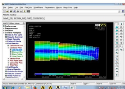
Gambar 6 Defleksi poros dengan berat kargo 1500 kg
