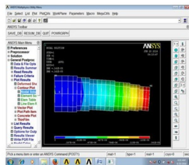
Gambar 6 Defleksi poros dengan berat kargo 1500 kg
