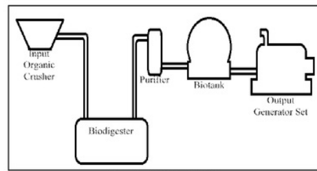
Gambar 3 siklus PLTG
