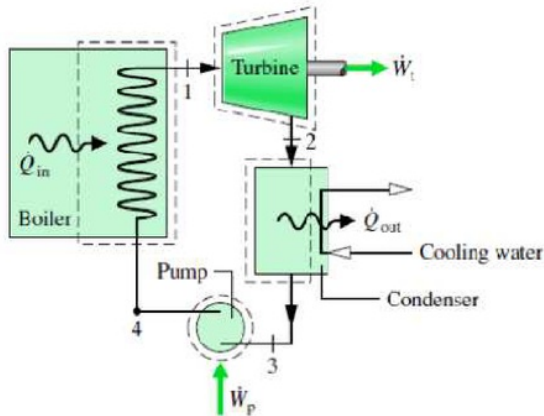
Gambar 2. Prinsip kerja sistem termodinamika.
