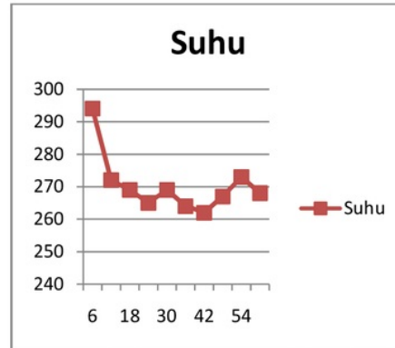
Gambar 7. Grafik hubungan temperatur pembakaran dan waktu.
