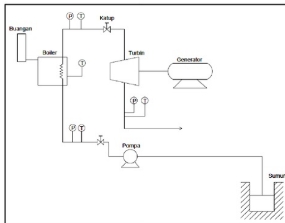
Gambar 5. Gambar mekanis rancangan prototype PLTU sekam padi.
