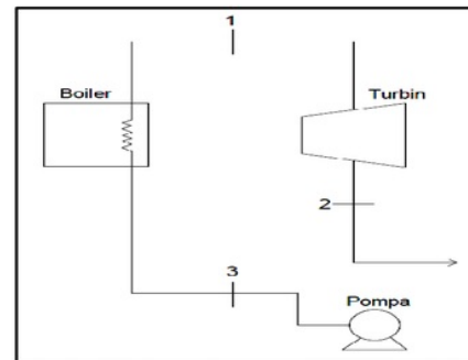
Gambar 8. Keadaan pada rancangan PLTU Sekam Padi.
