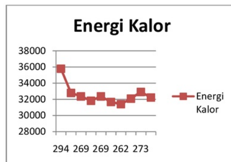
Gambar 9. Grafik hubungan energi kalor dan temperatur pembakaran.
