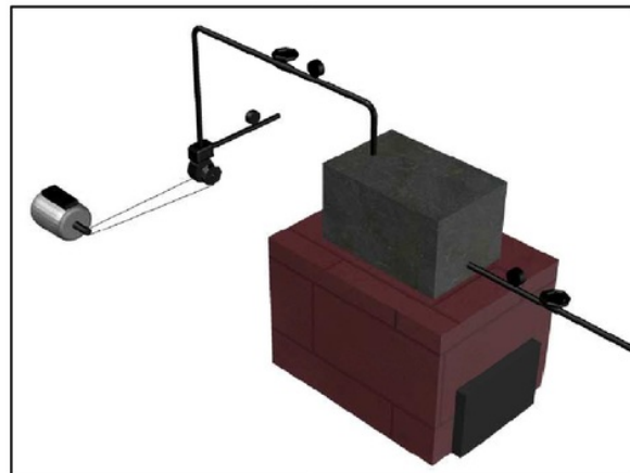
Gambar 4. Gambar desain rancangan prototype PLTU sekam padi.
