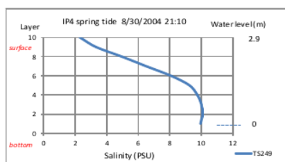
Gambar 6.Stratifikasi salinitas
