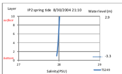
Gambar 5.Stratifikasi salinitas
