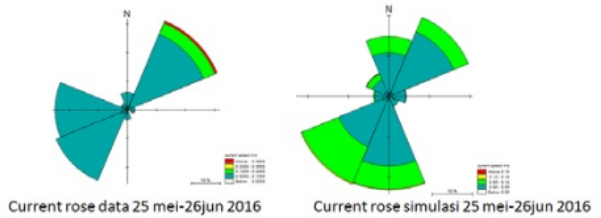
Gambar 6. Current Rose Data Dan Simulasi (pasut) Pada 25 Mei – 26 Juni 2016
