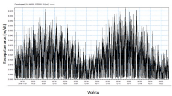
Gambar 12. Grafik Kecepatan Arus Pada Titik C
