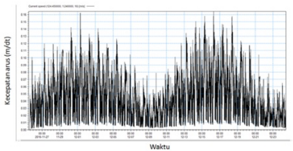
Gambar 10. Grafik Kecepatan Arus Pada Titik A
