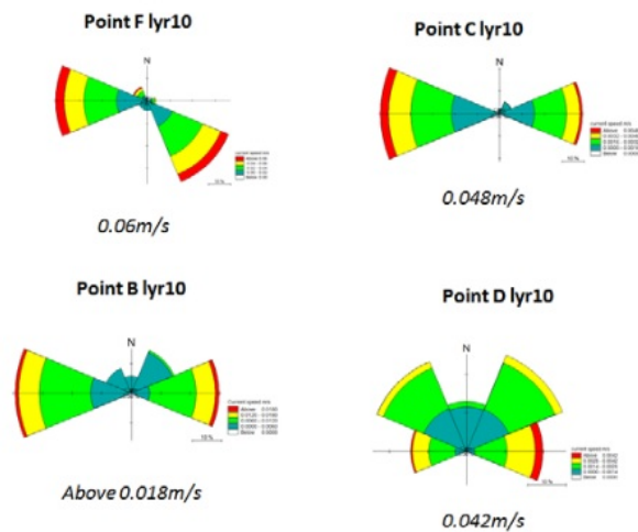
Gambar 7. Current Rose Titik F,C,B,D Akibat Pasang Surut
