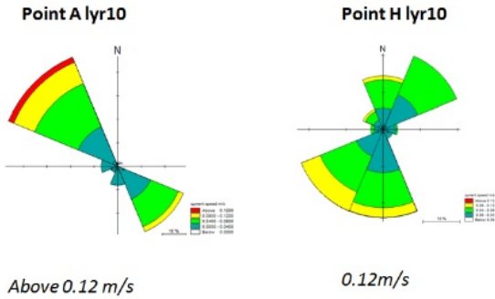
Gambar 8. Current Rose Titik A, H Akibat Pasang Surut
