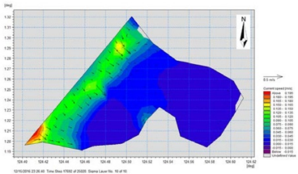
Gambar 9. Arus Dalam Kecepatan Dan Arah Pada Permukaan Air Saat Spring Tide
