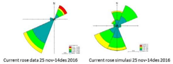
Gambar 5. Current Rose Data Dan Simulasi (pasut) Pada 25 Nov – 14 Des 2016
