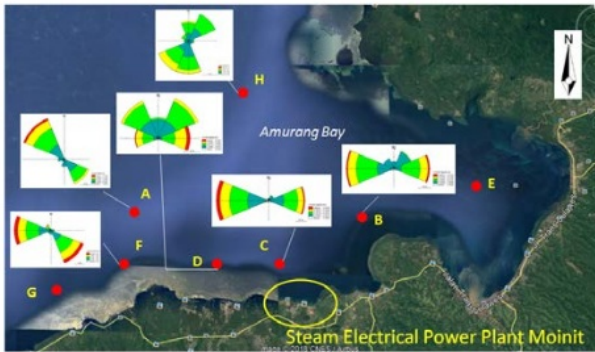
Gambar 3. Titik-titik Lokasi Studi dan Current-Rose Hasil Simulasi Tersebar Pada Teluk Amurang
