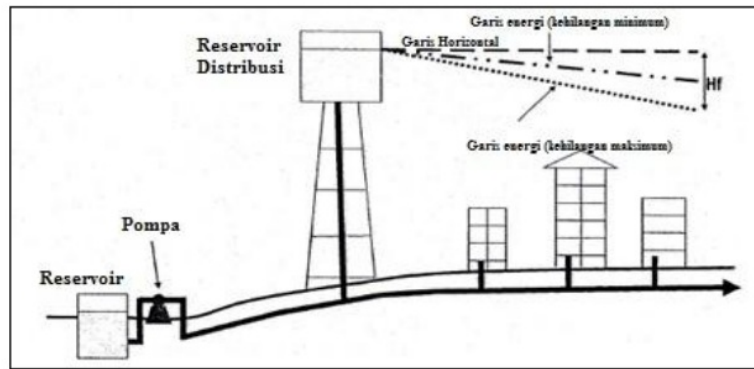
Gambar 5. Dual System Sumber : Tanudjaja, L. 2011
