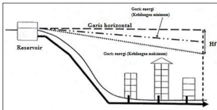
Gambar 3. Gravity System Sumber : Tanudjaja, L. 2011.
