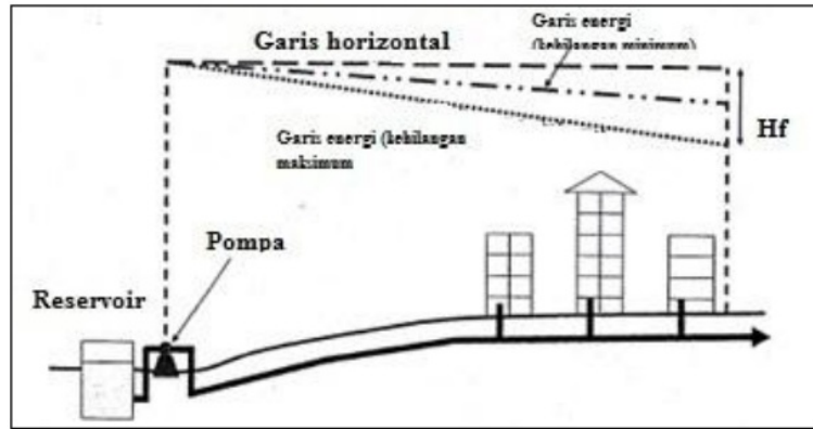
Gambar 4. Pumping System Sumber : Tanudjaja, L. 2011
