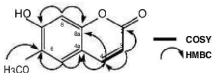
Gambar 2. Korelasi ^1\text{H} - ^1\text{H} COSY dan HMBC untuk senyawa 1
