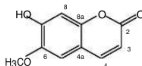
Gambar 1. Struktur kimia senyawa skopoletin
