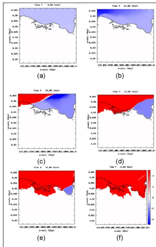
Gambar 8. Hasil simulasi penjaralan tsunami pada layer 5 pada menit Ke-0, (b) menit ke-11, (c) menit ke-16, (d) menit ke-17, (e) menit ke-18, (f) menit ke-19.
