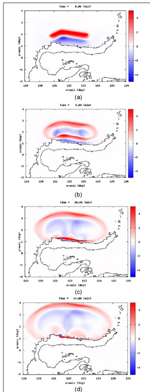
Gambar 6. Hasil simulasi penalaran tsunami di layer 1 pada (a) menit ke-0, (b) menit ke-5, (c) menit ke-10, (d) menit ke-14.
