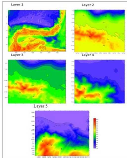
Gambar 5. Profil batimetri dan topografi area simulasi.
