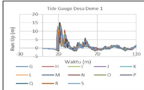
Gambar 11. Grafik ketinggian muka air laut hasil simulasi akibat tsunami pada setiap virtual tide gauge di Desa Deme 1.
