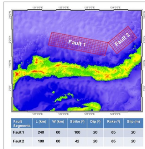
Gambar 3. Segmen sesar dan parameter bidang sesar yang digunakan dalam pemodelan tsunami
