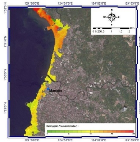
Gambar 7. Peta inundasi tsunami akibat gempa bumi berkekuatan M8,5 di Manado
