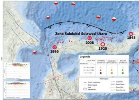
Gambar 1. Peta tatanan tektonik Pulau Sulawesi. Busur subduksi ditandai dengan garis tebal putus-putus dengan segitiga. Titik-titik merah adalah episenter gempa bumi. Lingkaran merah adalah gempa bumi yang pernah menimbulkan tsunami. Lingkaran merah-putih adalah bola fokal dari beberapa gempa besar yang pernah terjadi. (BMKG 2017)
