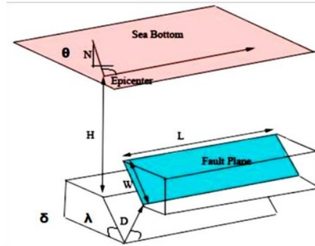
Gambar 2. Parameter-parameter sesar untuk input pemodelan sumber pembangkit tsunami.
