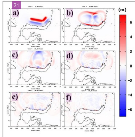
Gambar 5. Snapshot dan perjalanan tsunami pada menit ke 0 (a), 10 (b), 20 (c), 30 (d), 40 (e), dan 60 (f)
