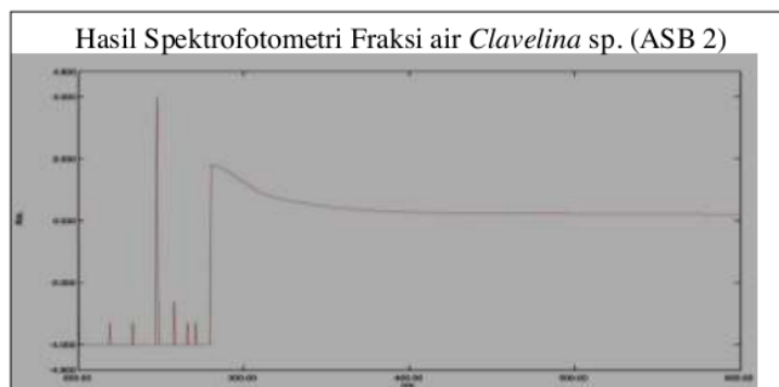
Gambar 8. Hasil Spektrofotometri Fraksi air Clavelina sp.
