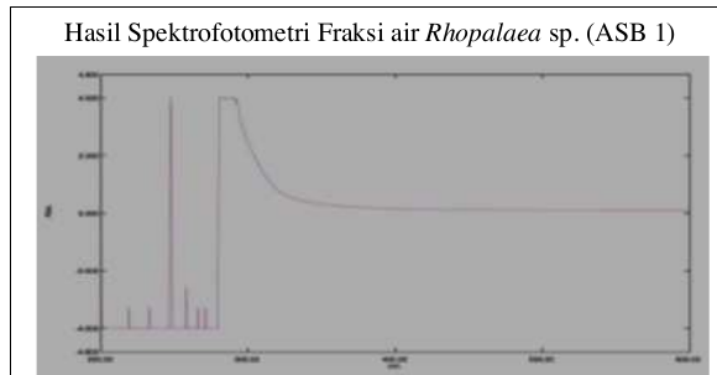
Gambar 7. Hasil Spektrofotometri Fraksi air Rhopalaea sp.
