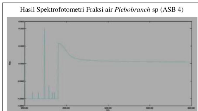
Gambar 10. Hasil Spektrofotometri Fraksi air Plebbranch sp.
