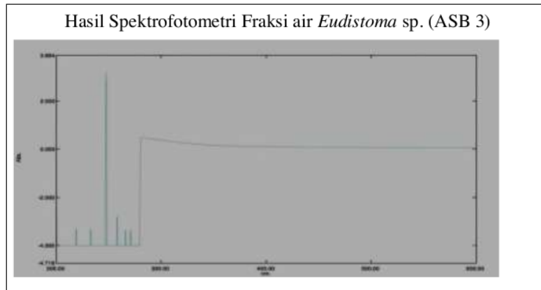
Gambar 9. Hasil Spektrofotometri Fraksi air Eudistoma sp.
