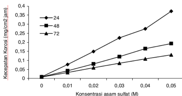
Gambar 1. Kurva pengaruh konsentrasi asam sulfat terhadap kecepatan korosi baja, perendaman selama 24, 48 dan 72 jam.
