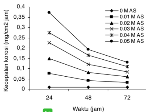
Gambar 2. Kurva pengaruh waktu perendaman terhadap kecepatan korosi baja dalam larutan asam sulfat 0,01; 0,02; 0,03; 0,04 dan 0,05 M.
