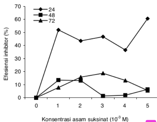
Gambar 5. Kurva efisiensi inhibisi asam suksinat pada korosi baja dalam larutan asam sulfat 0,05 M.
