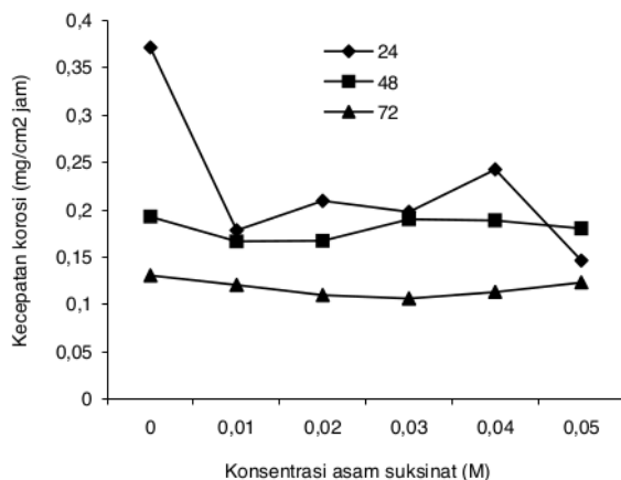
Gambar 3. Kurva pengaruh konsentrasi Asam Suksinat terhadap kecepatan korosi baja dalam larutan Asam Sulfat 0,05 M.
