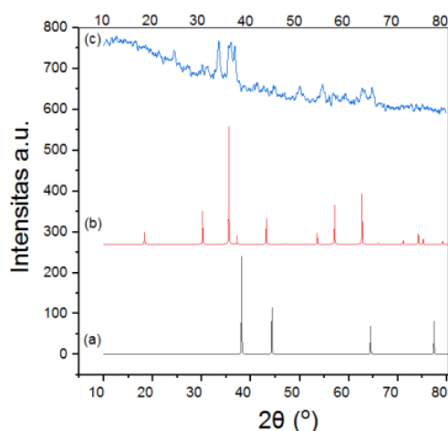
Gambar 3. Difraktogram nanopartikel Ag/ \text{CoFe}_2\text{O}_4 .
