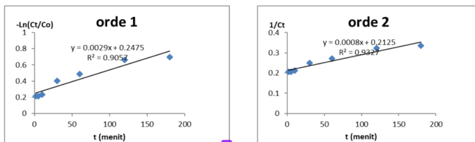
Gambar 4. Model kinetika fotodegradasi MB orde ke-1 dan orde ke-2 oleh komposit Ag_3PO_4/Ag/HAp dari tulang ikan terkalsinasi 800 °C.
