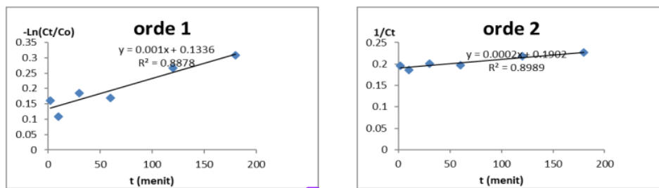
Gambar 5. Model kinetika fotodegradasi MB orde ke-1 dan orde ke-2 oleh komposit Ag_3PO_4/Ag/HAp dari tulang ikan terkalsinasi 1000 °C.
