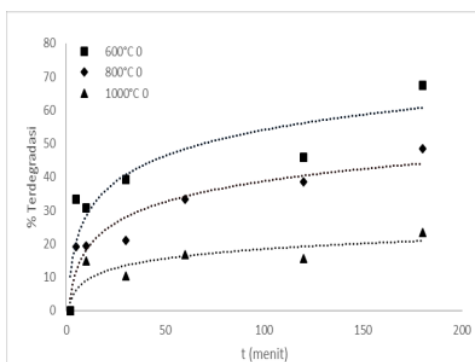
Gambar 2. Jumlah MB terdegradasi oleh komposit dari tulang ikan terkalsinasi pada berbagai suhu.
