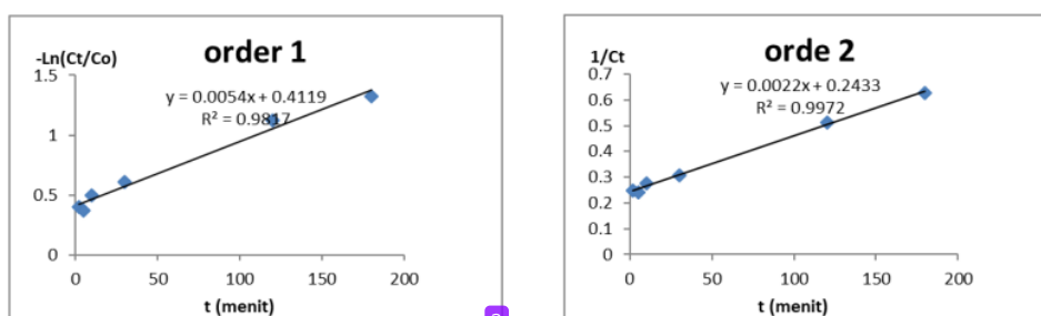
Gambar 3. Model kinetika fotodegradasi MB orde ke-1 dan orde ke-2 oleh komposit Ag_3PO_4/Ag/HAp dari tulang ikan terkalsinasi 600 °C.
