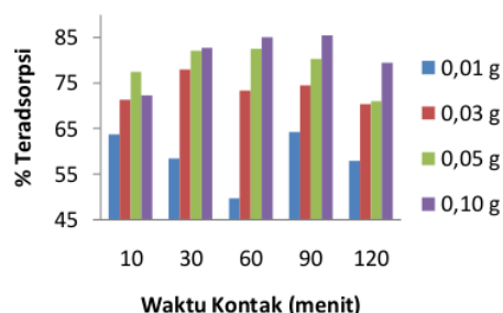
Gambar 2. Jumlah Zat Warna Methylene Blue yang Teradsorpsi (%) Karbon Aktif Kulit Pisang Goroho teraktivasi NaOH
