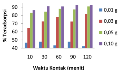
Gambar 1. Jumlah Zat Warna Methylene Blue yang Teradsorpsi (%) Karbon Aktif Kulit Pisang Goroho teraktivasi H 2 SO 4
