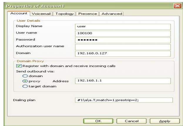
Gambar 12. Settingan pada softphone X-Lite
