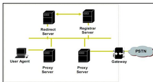
Gambar 5. Arsitektur SIP
