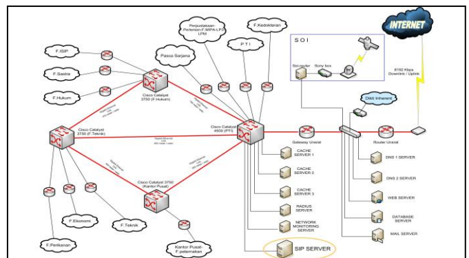
Gambar 8. Rancangan Jaringan VoIP dengan menggunakan SIP Server di Universitas Sam Ratulangi
