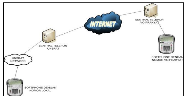
Gambar 13. Trunking dengan Voiprakyat
