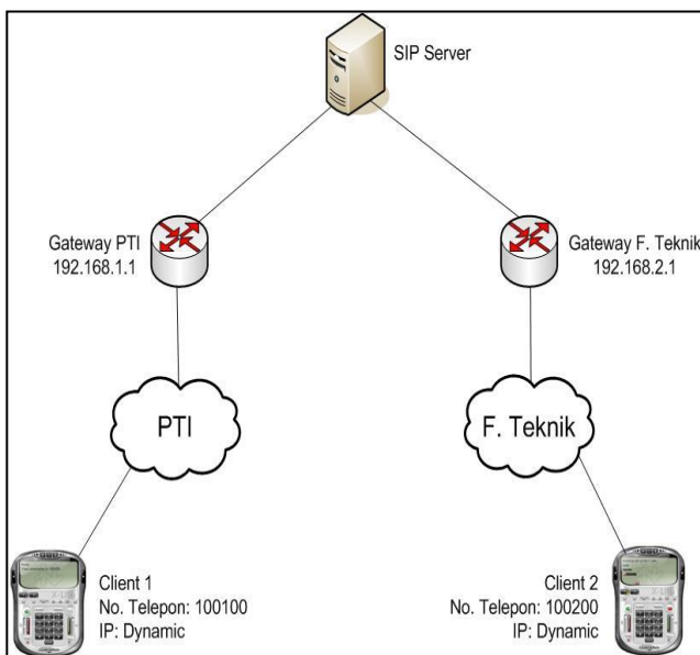
Gambar 11. Komunikasi Antara PTI - F. Teknik
